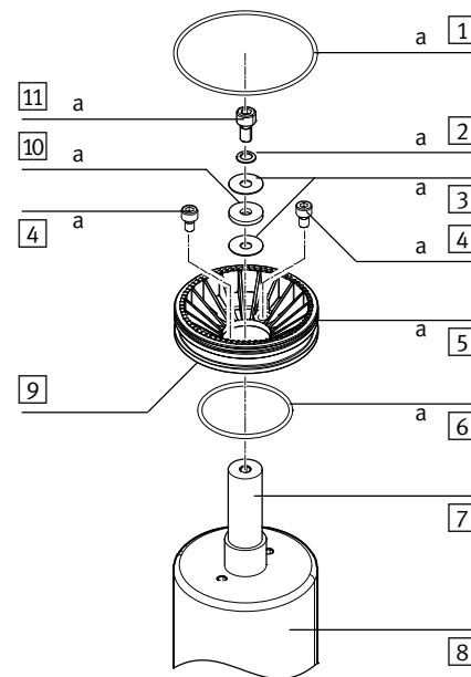
Fig. 4 : Montage de l'aimant (exemple)
