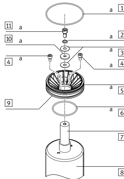
Fig. 4 : Magnet assembly (example)
