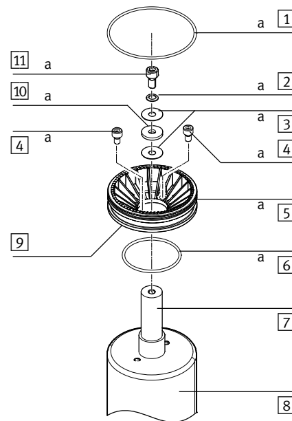
Fig. 4 : Magnetmontage (Beispiel)
